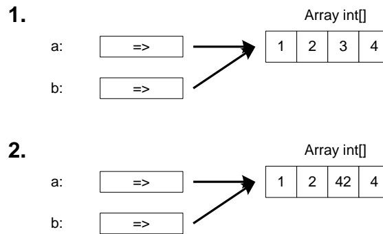
Abb. 10-1 : Referenz-Semantik bei Arrays
