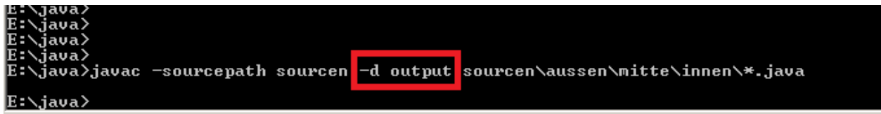
Abb. 4-21 : Der Java Compiler erzeugt den Byte-Code mit Trennung des Byte-Codes
