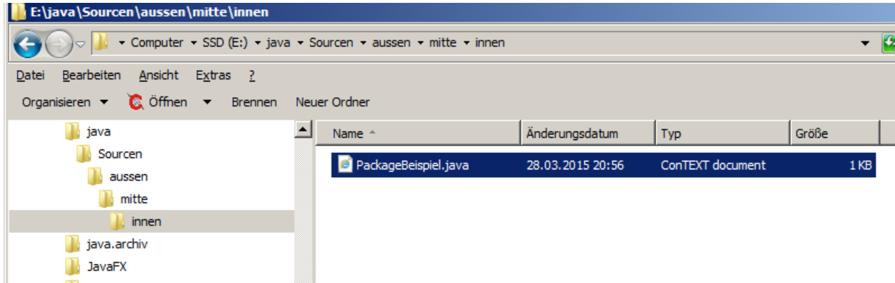
Abb. 4-13 : Verzeichnis-Struktur für das Package Beispiel
