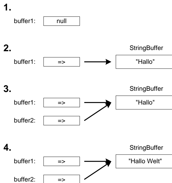
Abb. 5-2 : Referenz-Semantik
