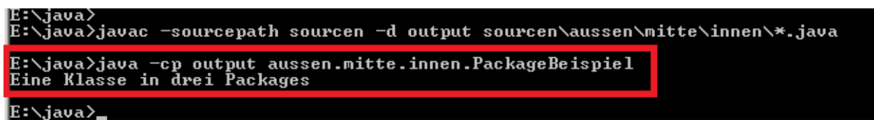
Abb. 4-23 : Korrekte Ausführung des Package Beispiels mit Trennung des Byte-Codes
